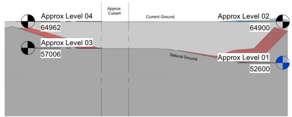
3 Section 3 1 : 500
