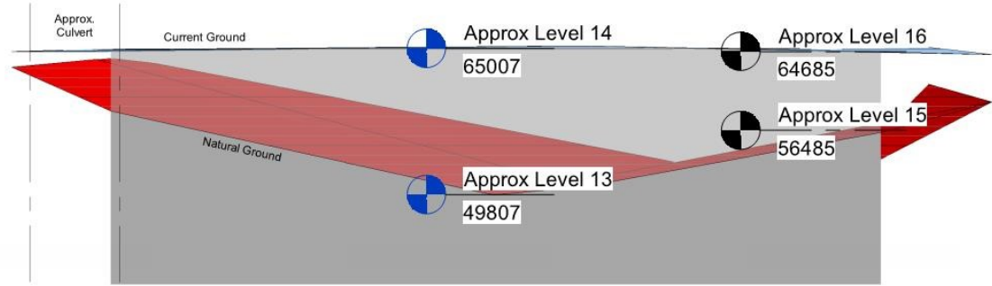
1 Section 1 1 : 500
