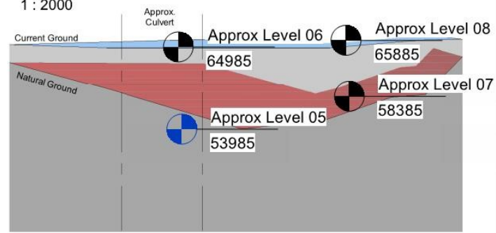
4 Section 4 1 : 500
